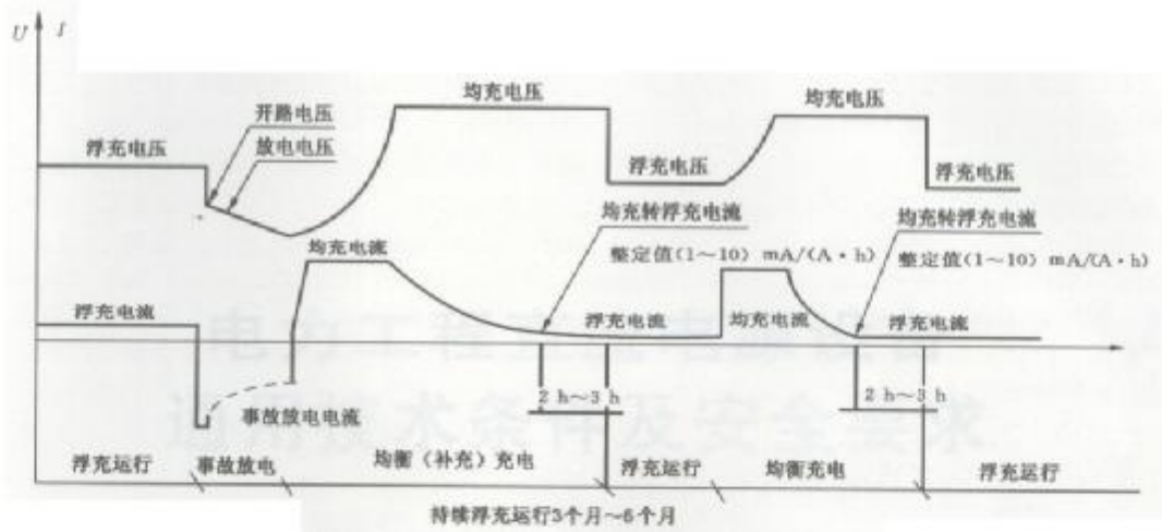
图 C.1 直流电源设备充放电特性示意图
